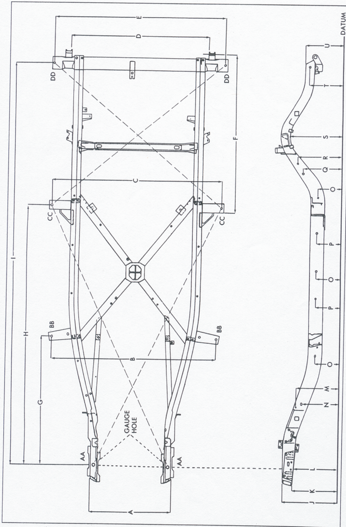
Fig. 1—Frame Dimensions
